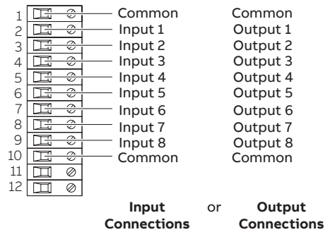
Digital Input/Output Module
